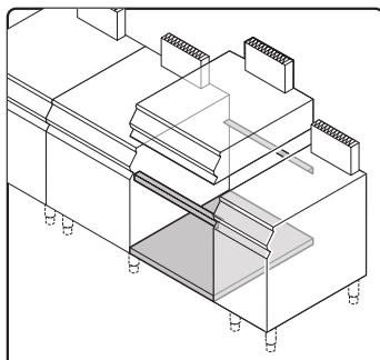
соединительные элементы для мостового соединения
